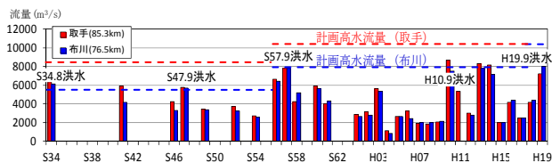
図-4 年最大流量
