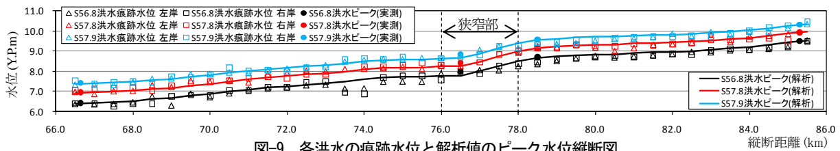
図-9 各洪水の痕跡水位と解析値のピーク水位縦断面図
